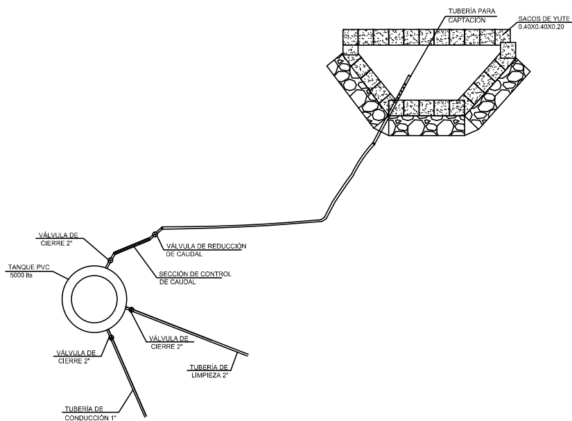
Figura 8-30 Esquema Puntos de Captación
