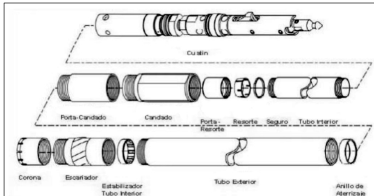
Figura 8-14 Sarta de perforación y sus componentes.
