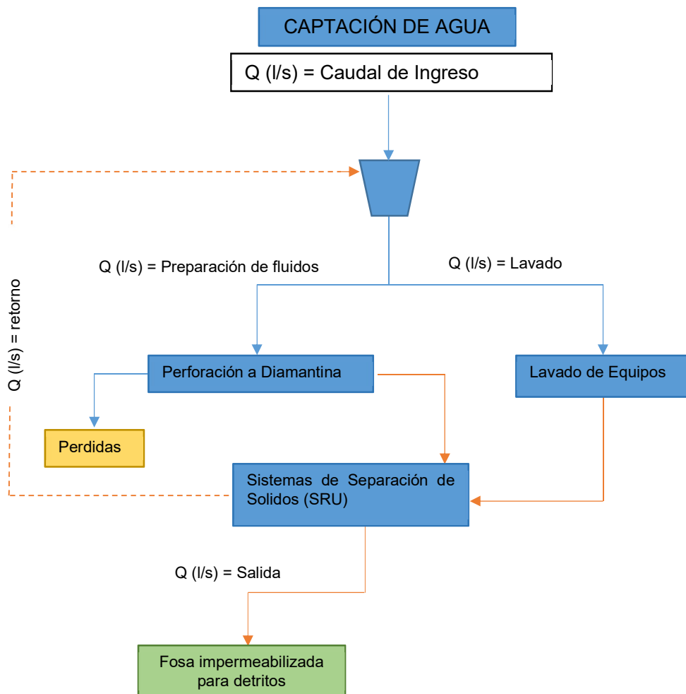
Figura 8-33 Balance de agua para proceso de perforación
