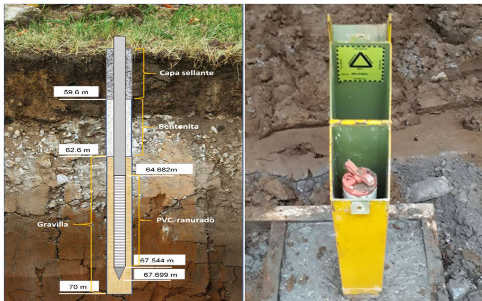
Figura 8-11 Estructura de un Piezómetro.
