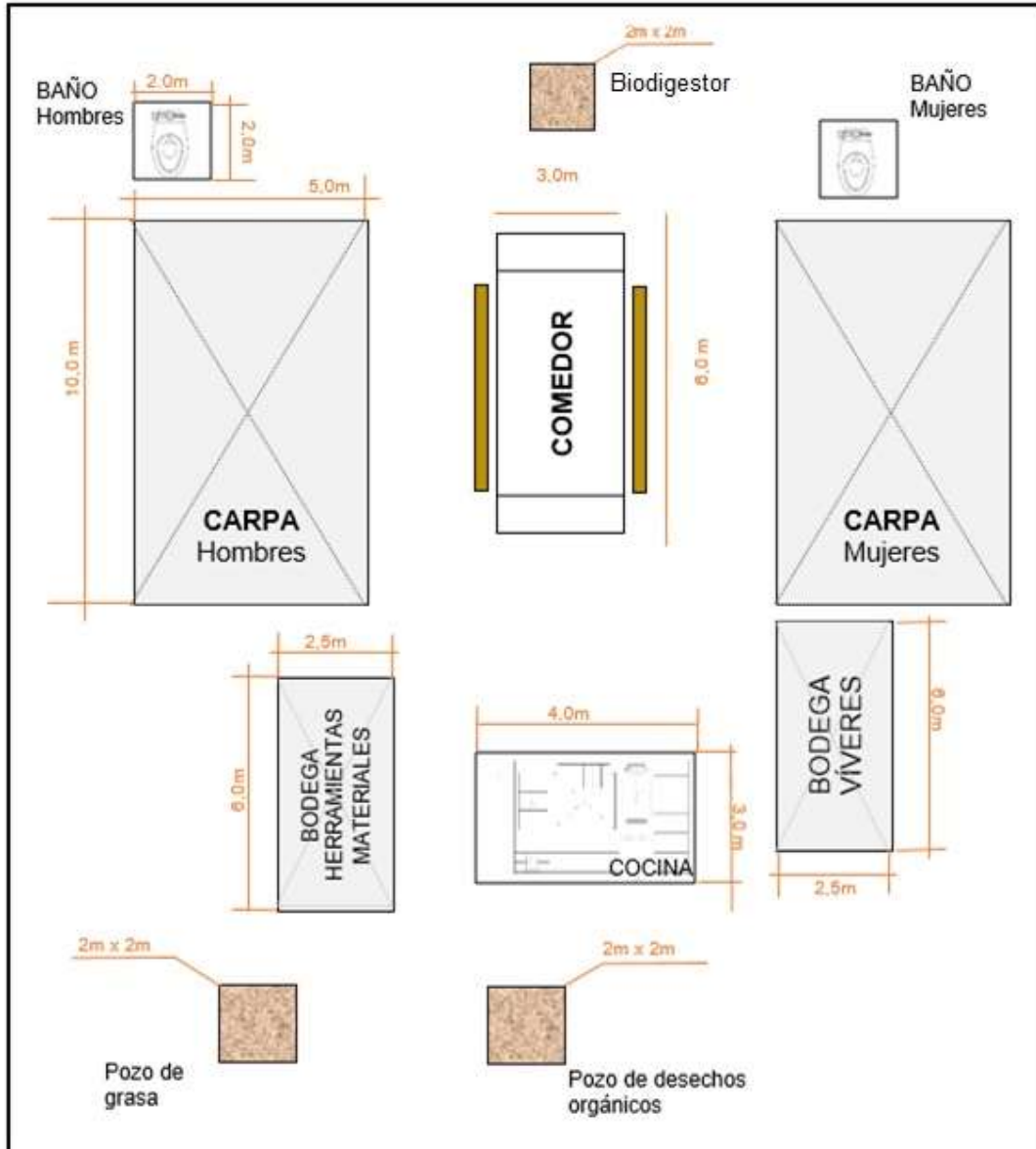
Figura 8-7 Esquema Referencial de Implantación de Campamentos Flotantes
