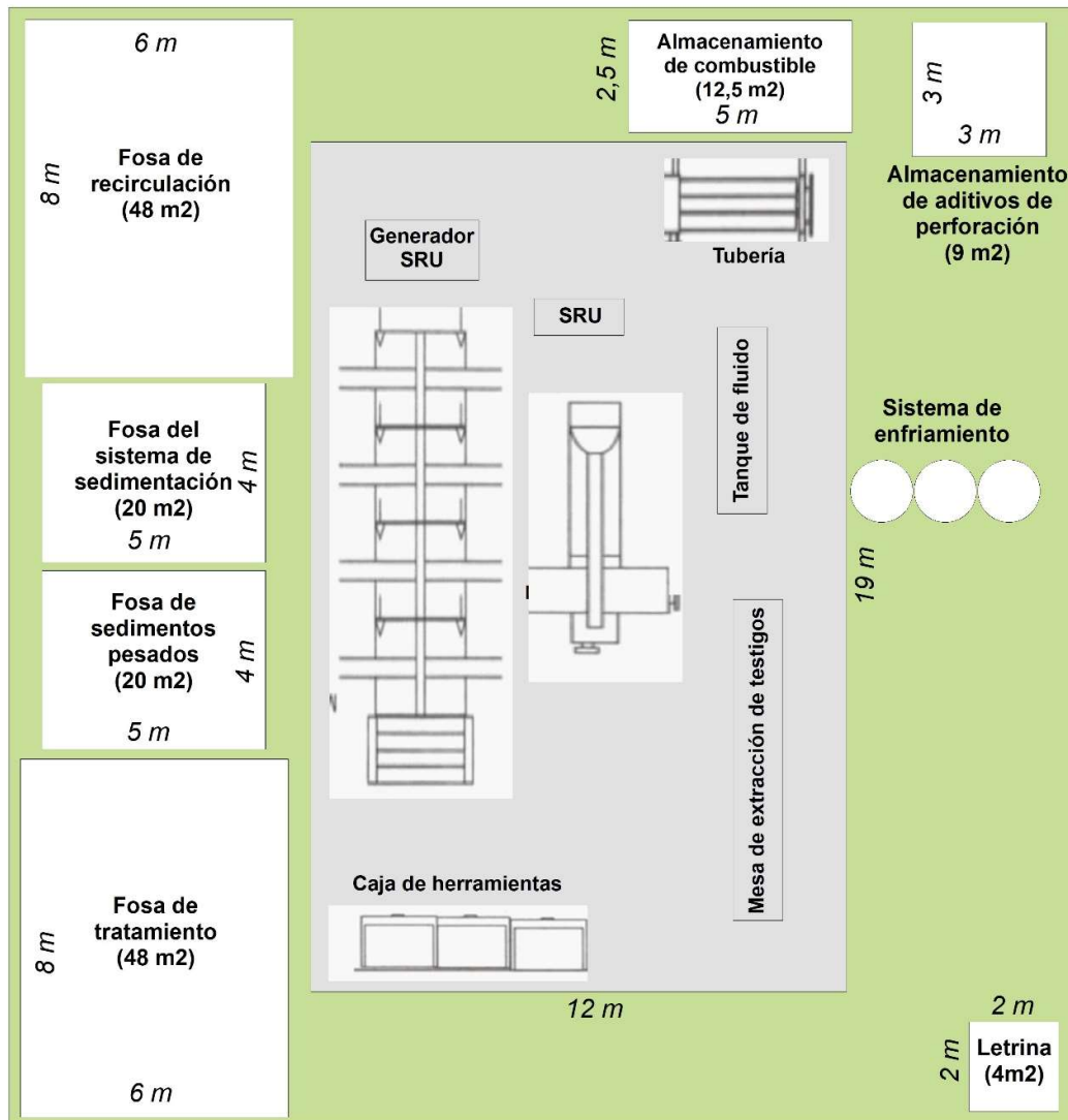
Figura 8-9 Implantación Referencial de Plataforma para Taladros Portables
