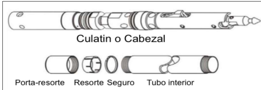
Figura 8-19 Core Barril y sus componentes.
