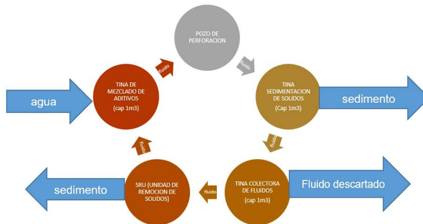
Figura 8-32 Diagrama de Flujo
