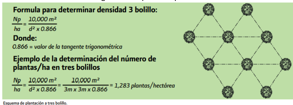
Figura 16. Esquema de plantación a tres bolillos
