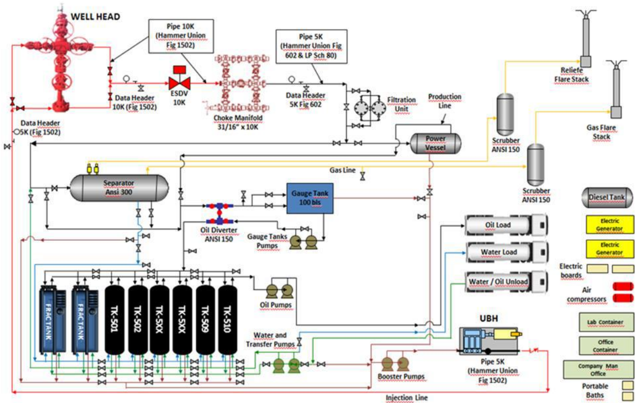
Figura 22. Diagrama del proceso de pruebas de producción
