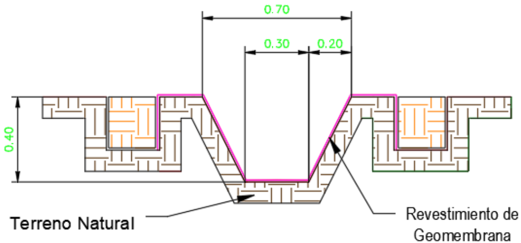
Figura 4. Diseño propuesto para cunetas perimetrales de geomembrana
