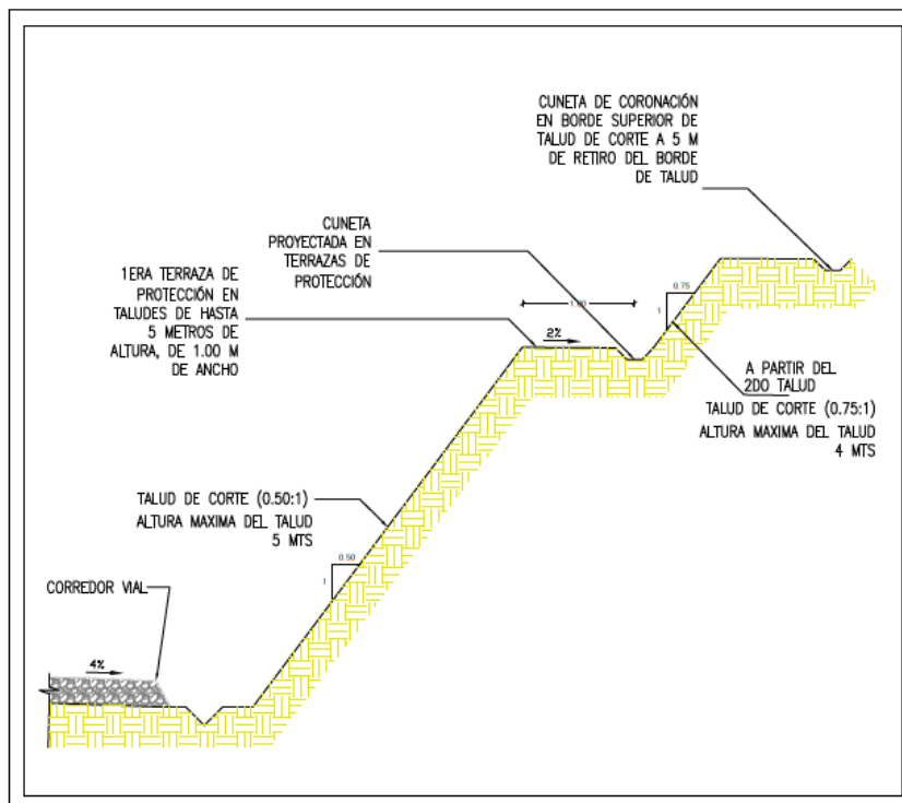
Figura 14. Diseño propuesto para cunetas de coronación
