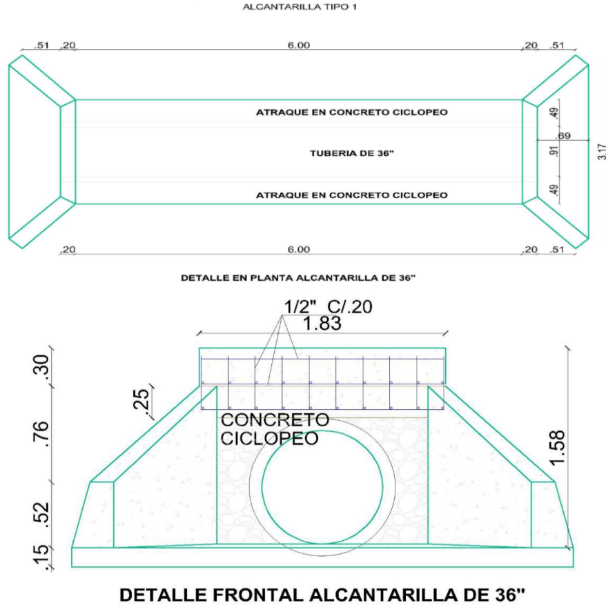
Figura 13. Diseño de alcantarilla tipo
