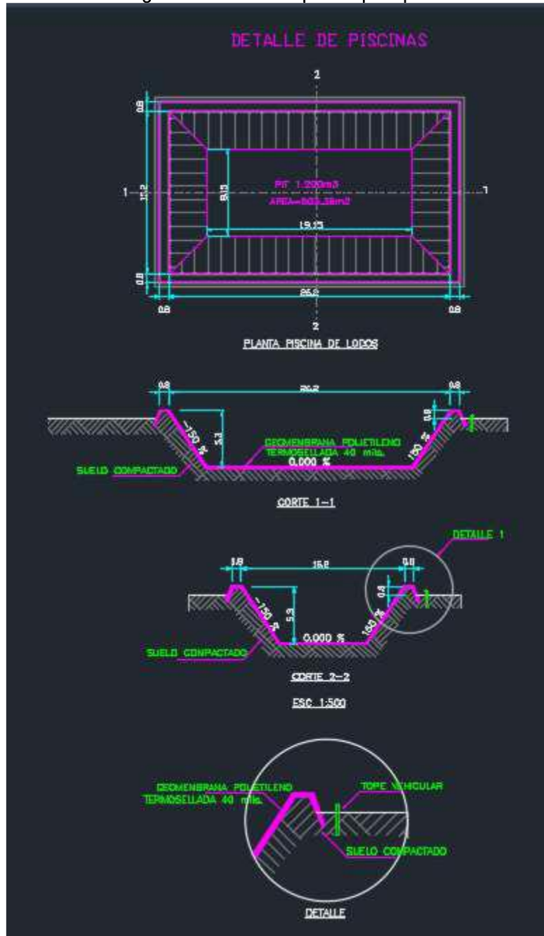
Figura 21. Diseño Propuesto para piscinas
