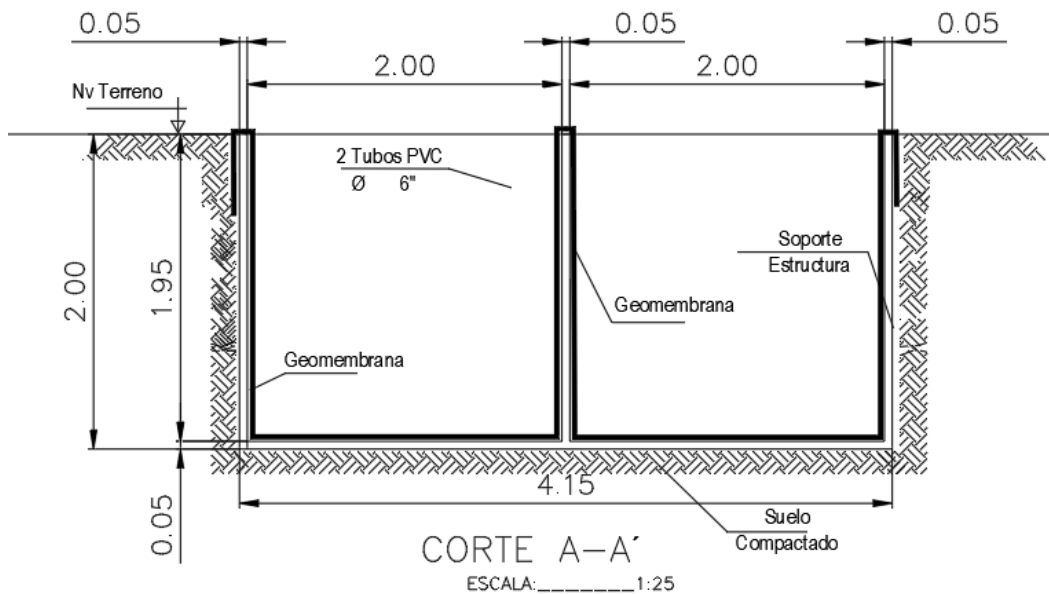
Figura 5. Diseño de Trampa de Grasa API y desarenador
