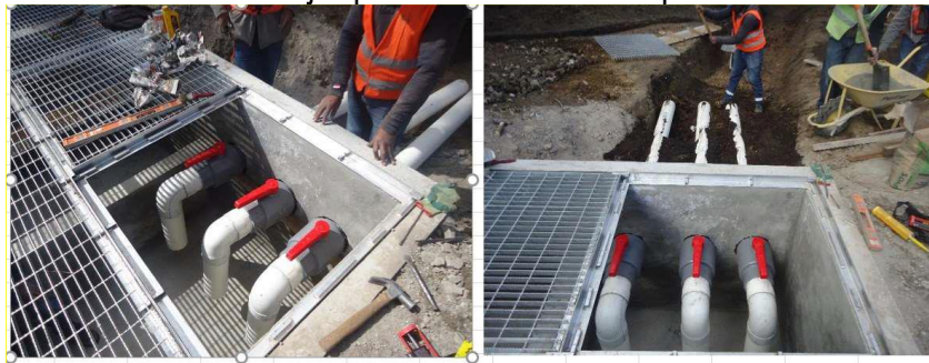
Foto 11. Ejemplos de instalación Trampas API
