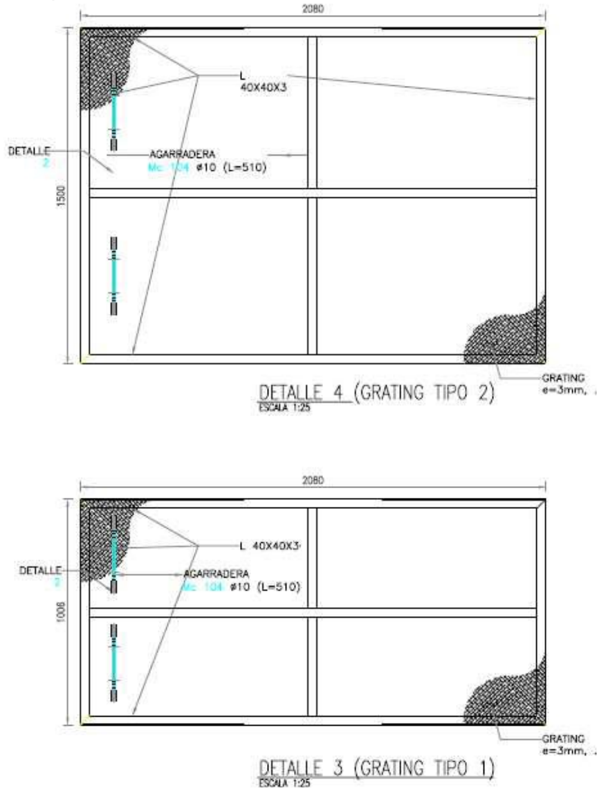
Figura 6. Detalles de cubierta para la Trampa de Grasas API
