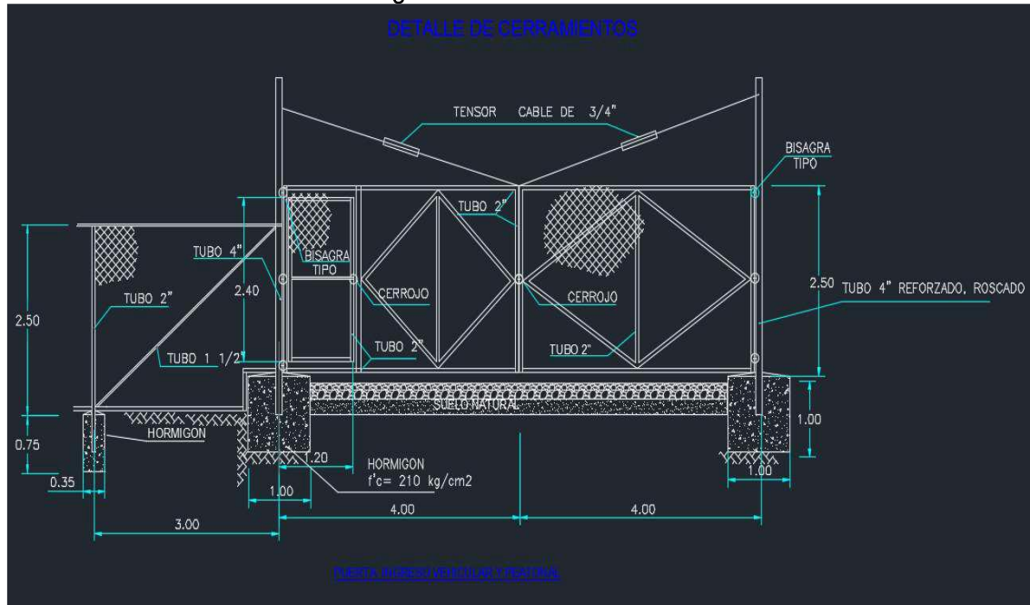
Figura 8. Diseño de Cerramiento Perimetral
