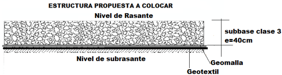
Figura 3. Estructura Propuesta a colocar para las plataformas y accesos.
