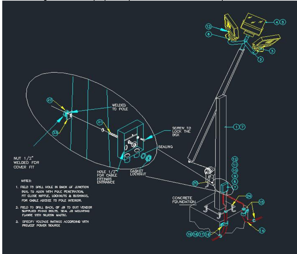
Figura 9. Diseño propuesto para sistema de iluminación perimetral
