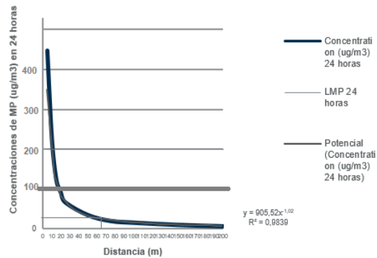
Figura 10 Concentración de MP (ug/m 3 ) en 24 horas
