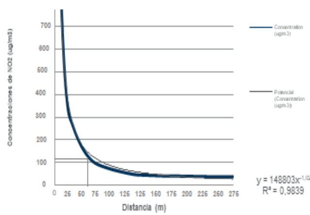
Figura 14 Concentración de NO 2 (ug/m 3 ) en 1 hora
