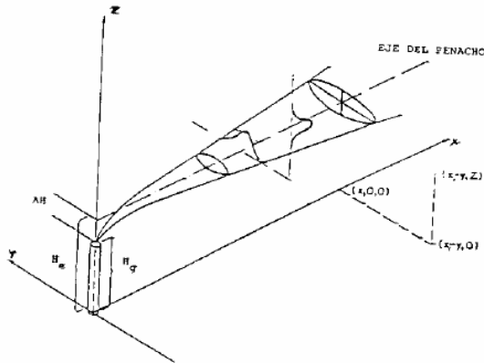
Figura 8 Modelo gaussiano para dispersión de contaminantes atmosféricos
