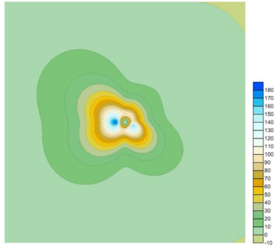
Figura 12 Resultados gráficos de las concentraciones horarias de Dióxido de Azufre (SO 2 ) (µg/m 3 ) entregados por el modelo de dispersión de gases
