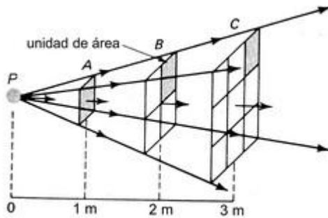
Figura 2 Representación de la Ley del cuadrado de la distancia
